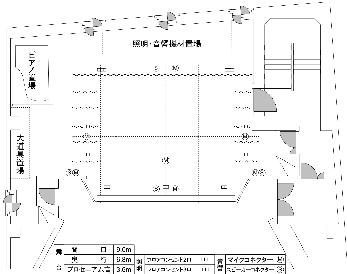
〔常陽藝文ホール舞台平面図〕
